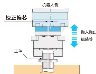
校正机器人搬运时的偏心
